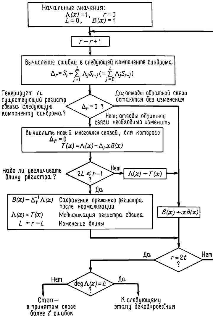
Рис. 7.5. Алгоритм Берлекэмпа—Мессе,
