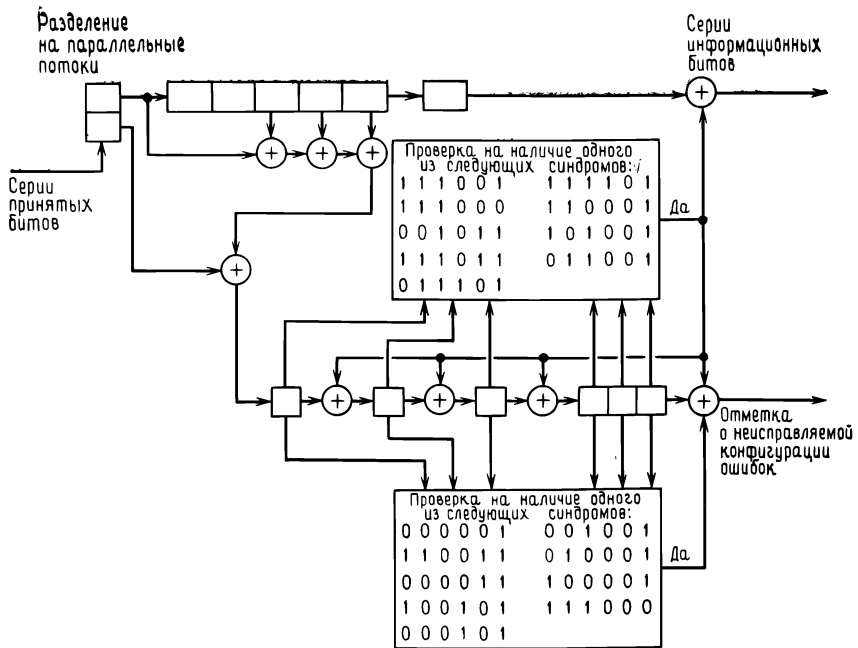
Рис. 12.20. Другой декодер для сверточного (12, 6)-кода.
