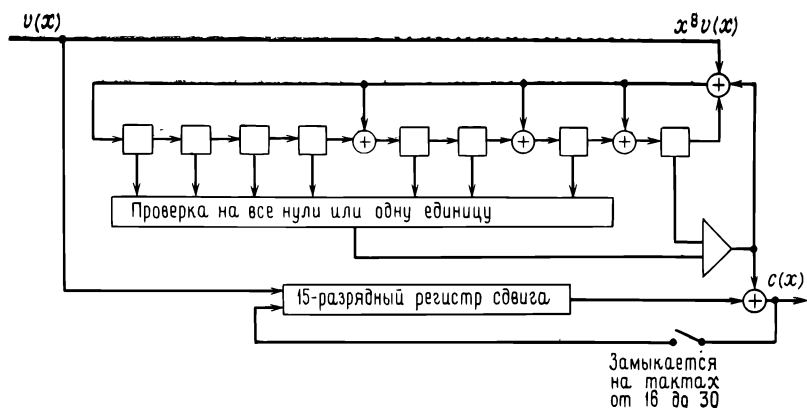
Рис. 6.24. Декодер с вылавливанием ошибок для (15, 7)-кода БЧХ.
