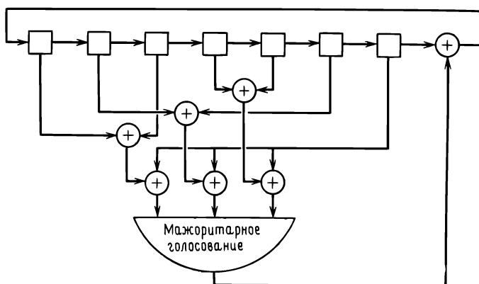
Рис. 13.1. Мажоритарный декодер для симплексного (7, 3)-кода.
