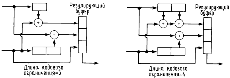
Рис. 12.9. Кодеры для двух сверточных кодов со скоростью 2/3.
