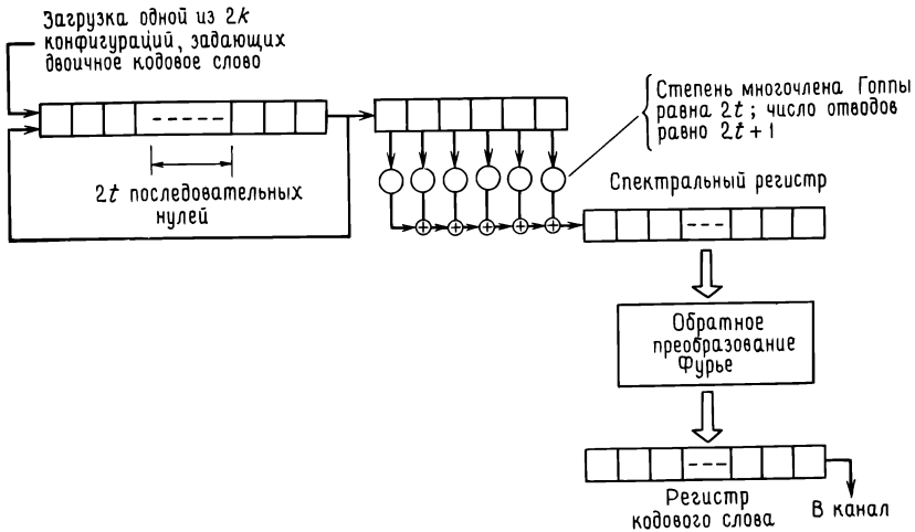
Рис. 8.11. Частотный кодер для кода Гоппы.
