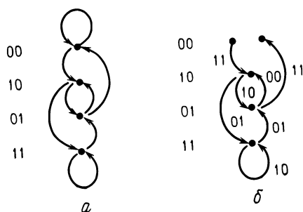
Рис. 14.5. Диаграмма состояний для сверточного (6, 3)-кода.
