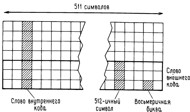
Рис. 7.10. Каскадный код, построенный из (511, 505)- и (7, 3)-кодов Рида—Соломона.
