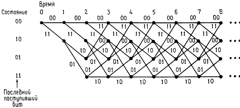
Рис. 12.5. Решетчатая диаграмма сверточного (6, 3)-кода.
