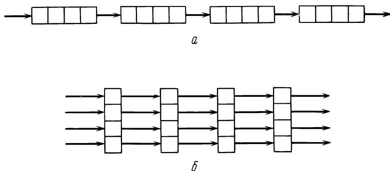
Рис. 6.3. Построенные из двоичных компонентов регистры сдвига для поля из 16 элементов. a — последовательное исполнение; б — параллельное исполнение.
