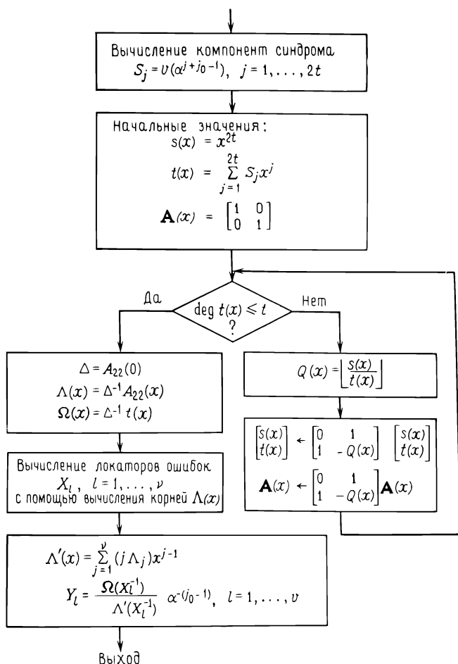
Рис. 7.8. Декодирование кодов БЧХ при помощи алгоритма Евклида.
