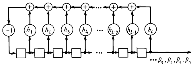
Рис. 6.6. Устройство циклического сдвига многочлена.
