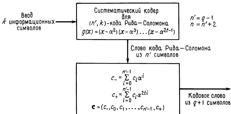
Рис. 8.7. Систематический кодер для расширенного кода Рида—Соломона.
