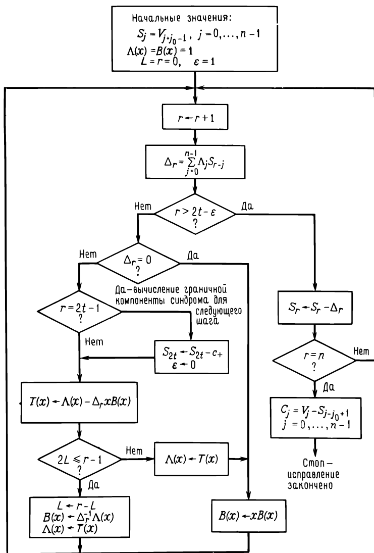
Рис. 9.5. Декодер для расширенного на один символ кода Риды—Соломона.
