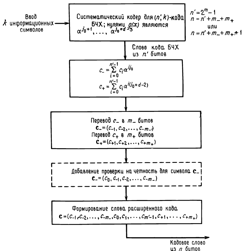
Рис. 8.10. Систематический кодер для расширенного кода БЧХ.
