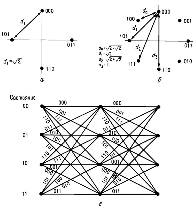
Рис. 15.6. Простой пример кодирования. a — четверичный набор ФТ-модулированных сигналов при отсутствии кодирования; б — восьмеричный набор ФТ-модулированных сигналов; в — решетка для сверточного (6, 4)-кода.
