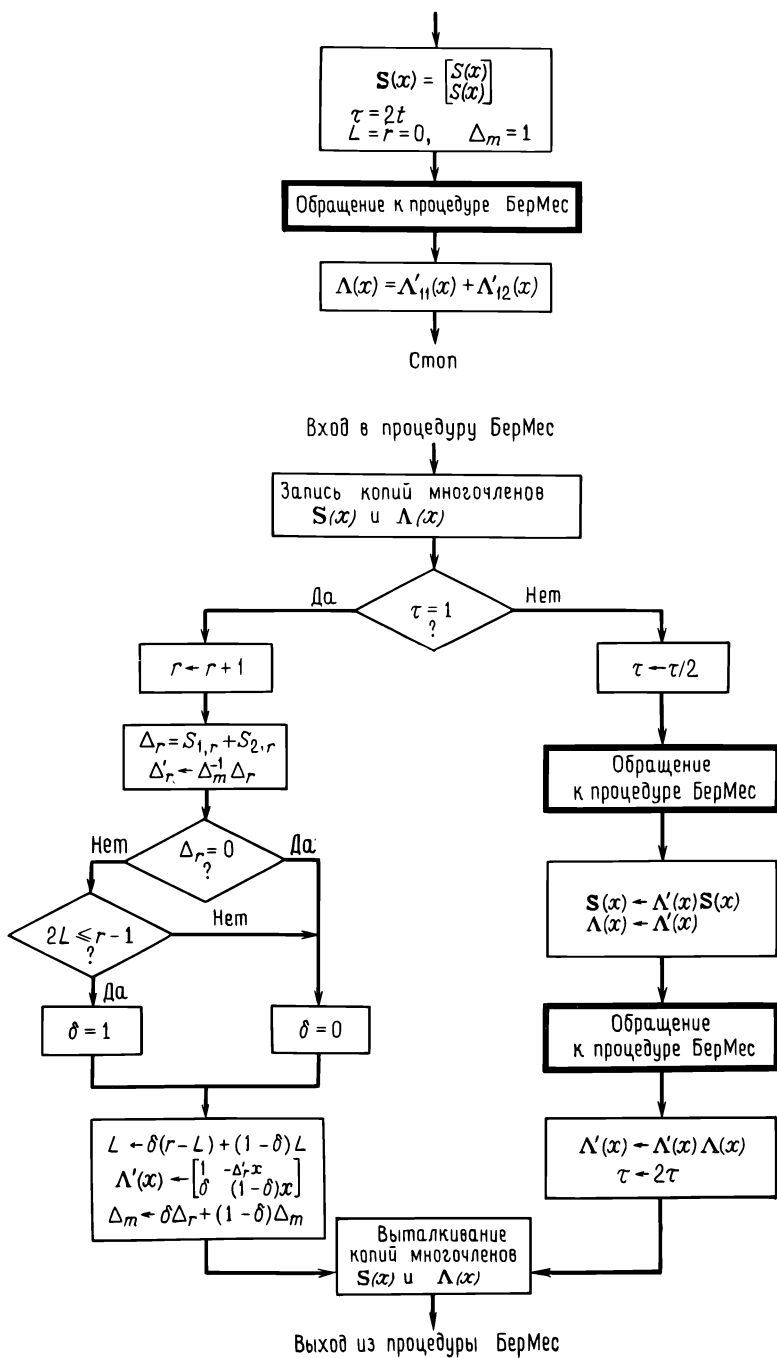
Рис. 11.8. Процедура БерМес.
