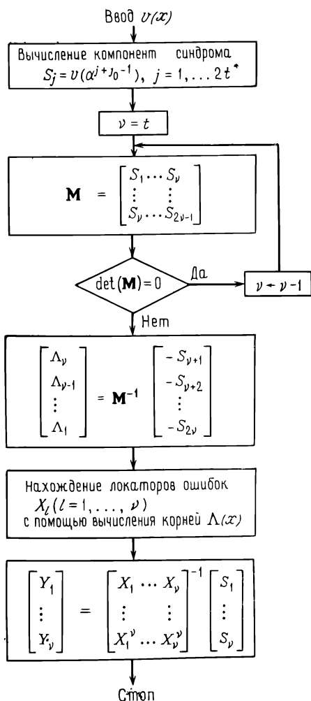
Рис. 7.1. Декодер Питерсона—Горенштейна—Цирлера.
