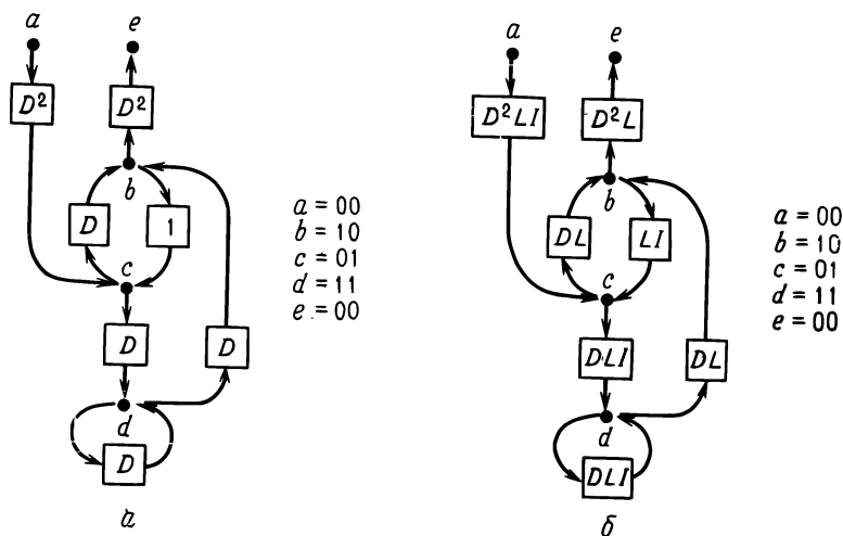
Рис. 14.6. Модифицированная диаграмма состояний для сверточного (6, 3)-кода. a — с переменной D , подсчитывающей задержку; b — с переменными D , L и I , подсчитывающими соответственно задержку, число кадров и число единиц на входе.
