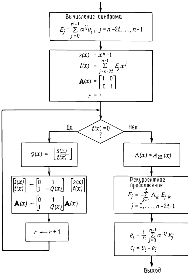
Рис. 9.3. Декодер для кодов БЧХ, основанный на алгоритме Евклида.
