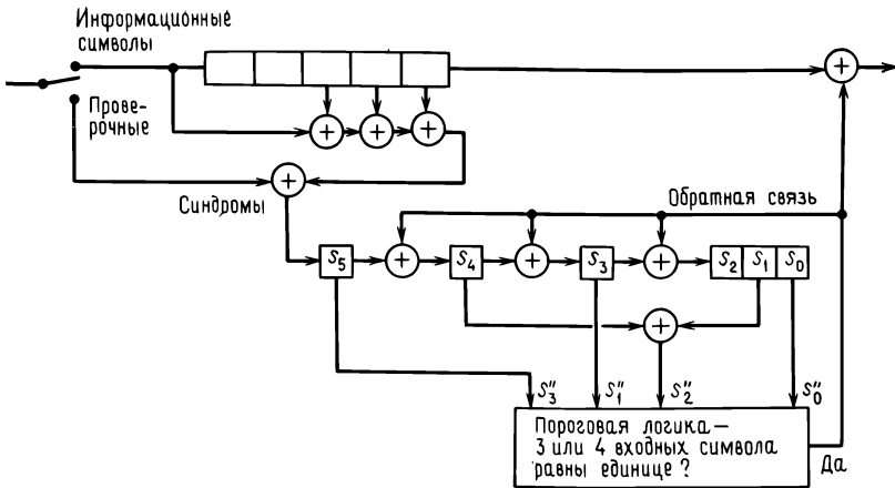
Рис. 13.5. Другой мажоритарный декодер.
