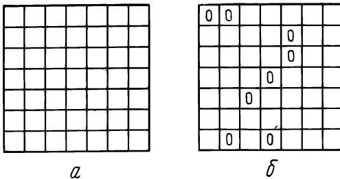
Рис. 10.3. Двумерный спектр над GF(8) . a — спектр без ограничений; b — спектр с ограничениями.
