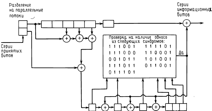
Рис. 12.19. Декодер для сверточного (12, 6)-кода.
