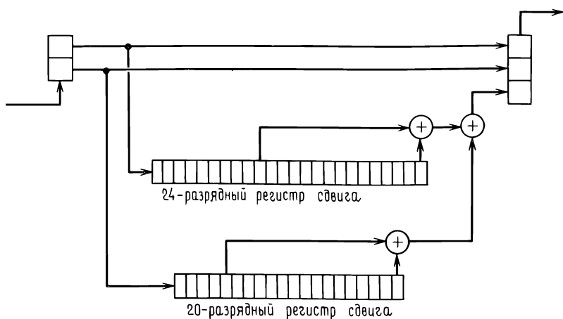
Рис. 12.21. Кодер для (72, 48)-кода Ивадаре.
