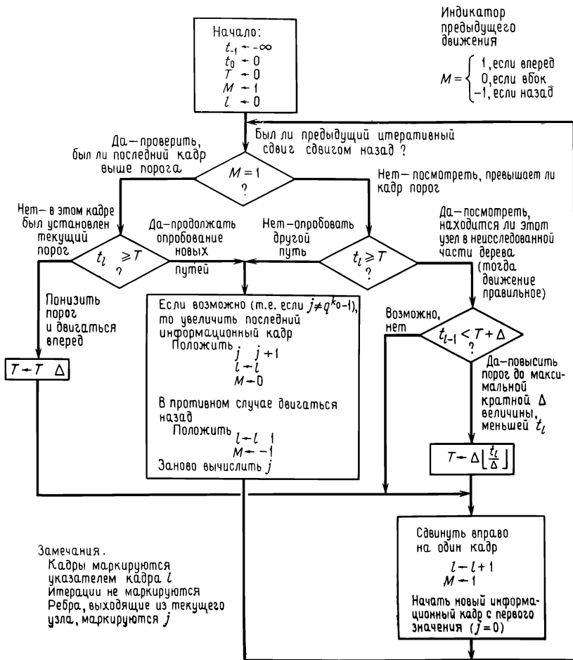
Рис. 12.27. Развернутый алгоритм Фано.
