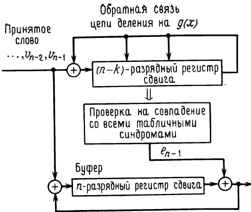
Рис. 6.18. Декодер Меггитта.
