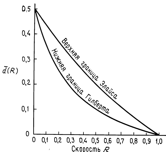
Рис. 14.7. Некоторые известные границы функции \bar{d}(R) при q = 2 .
