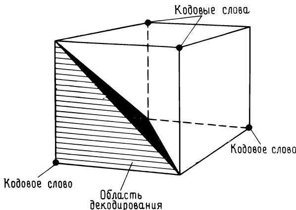
Рис. 15.4. Область декодирования по ОМР-алгоритму для двоичного (3, 2)-кода.
