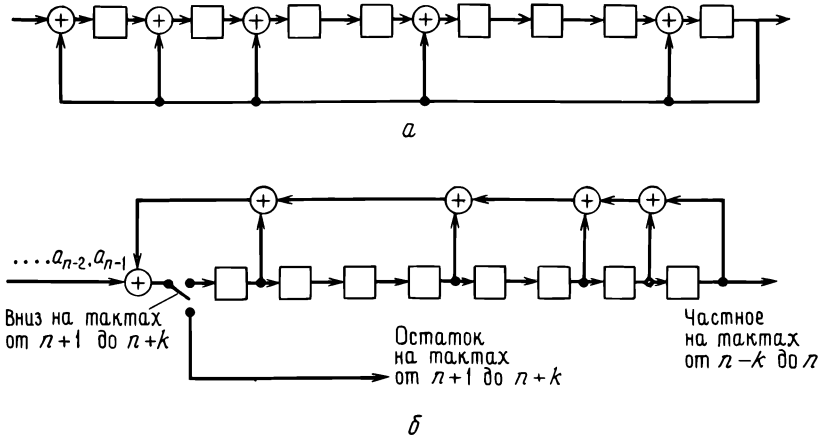
Рис. 6.12. Два устройства деления на многочлен x^8 + x^7 + x^4 + x^2 + x + 1 .
