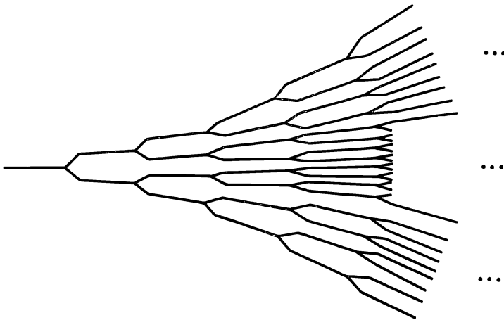
Рис. 12.6. Дерево для двоичного древовидного кода со скоростью 1/2.
