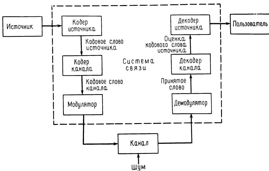
Рис. 1.1. Блок-схема цифровой системы связи.
