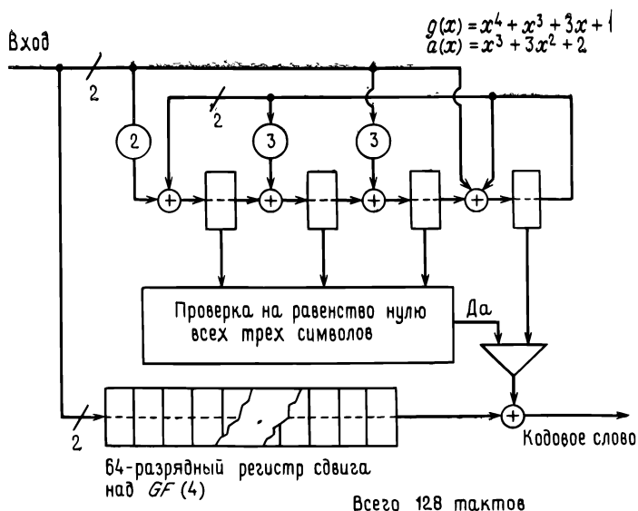
Рис. 6.31. Декодер Меггитта для (64, 60) -кода Хэмминга над GF(4) .
