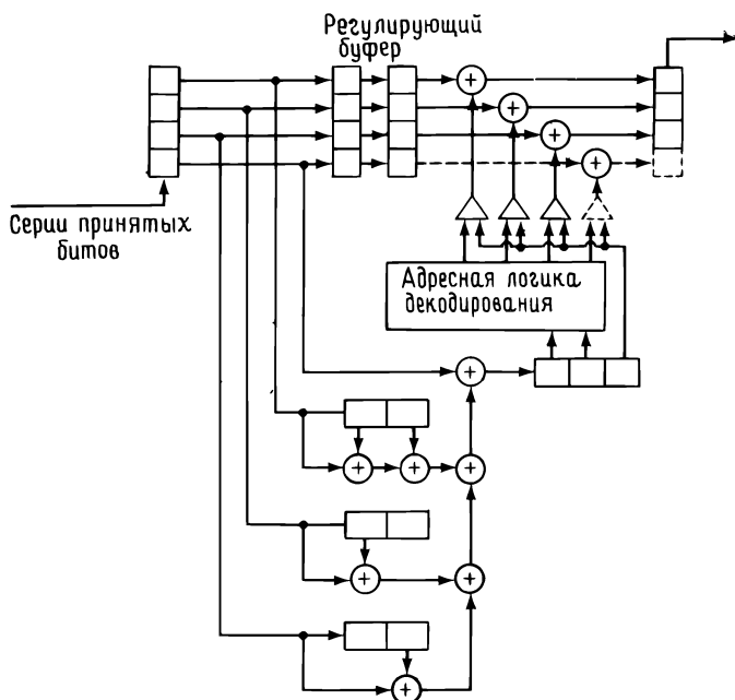
Рис. 12.14. Декодер для (12, 9)-кода Вайнера—Эша.
