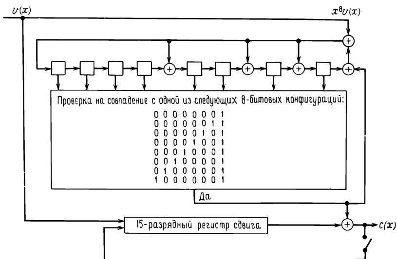
Рис. 6.23. Другой декодер Меггитта для (15, 7)-кода БЧХ.
