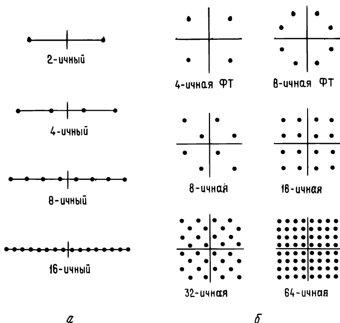
Рис. 15.1. Некоторые наборы сигналов. a — вещественные модуляционные алфавиты; б — комплексные модуляционные алфавиты (фазовая телеграфия).
