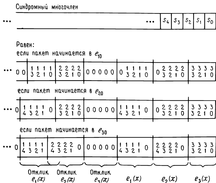
Рис. 12.22. Структура синдрома для (72, 48)-кода Ивадаре.
