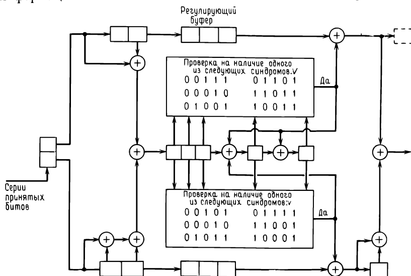
Рис. 12.16. Декодер для сверточного (6, 3)-кода.
