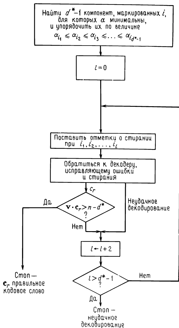
Рис. 15.5. ОМР-алгоритм.
