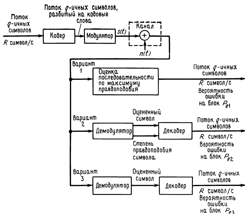
Рис. 15.3. Возможные варианты приемника.
