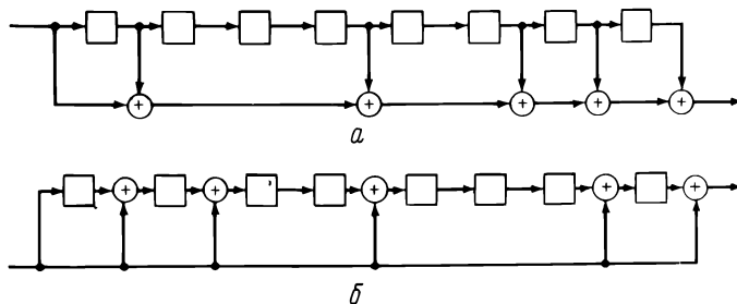
Рис. 6.10. Два устройства умножения на многочлен x^8 + x^7 + x^4 + x^2 + x + 1 .
