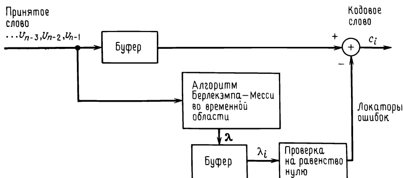
Рис. 9.6. Временной декодер для двоичного кода БЧХ.
