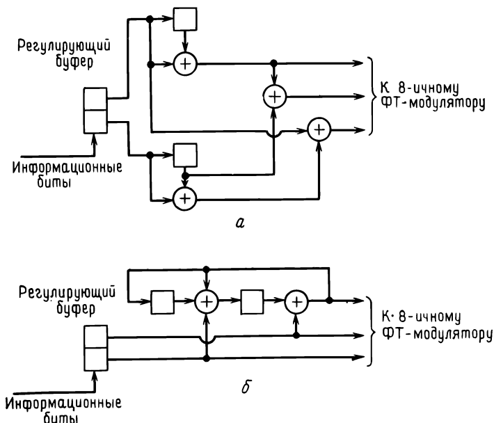
Рис. 15.7. Кодеры для сверточного (6, 4)-кода, а — кодер с регистром сдвига, не использующий обратную связь; б — кодер с регистром сдвига, использующий обратную связь.
