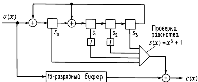
Рис. 6.19. Декодер Меггитта для (15, 11)-кода Хэмминга.
