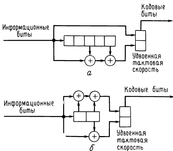
Рис. 12.3. Примеры сверточных кодеров. a — кодер для двоичного сверточного (12, 6)-кода; б — кодер для двоичного сверточного (6, 3)-кода.
