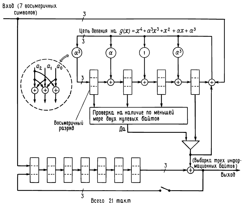
Рис. 6.27. Вылавливание ошибок для (7, 3)-кода Рида—Соломона.
