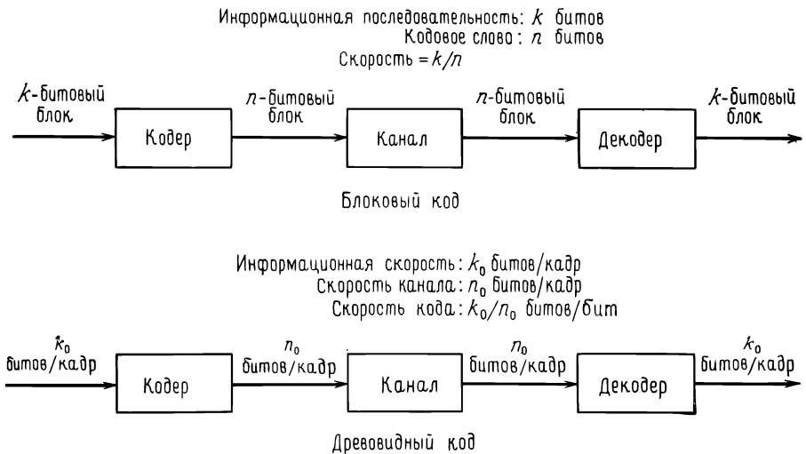
Рис. 1.2. Основные классы кодов.
