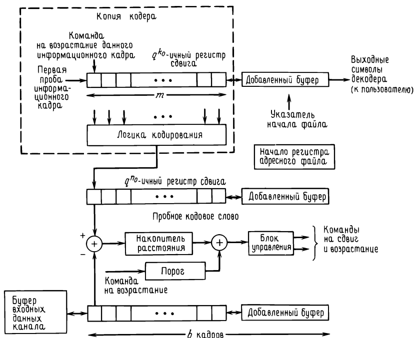
Рис. 12.26. Реализация алгоритма Фано в виде регистра сдвига.
