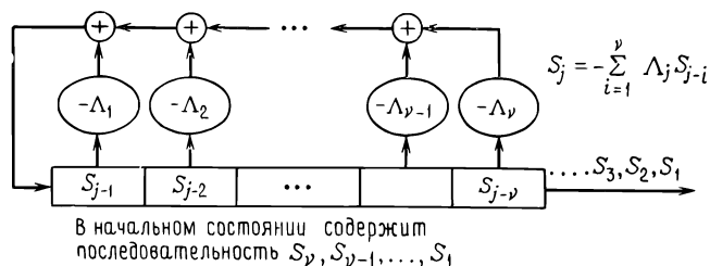
Рис. 7.2. Многочлен локаторов ошибок в цепи регистра сдвига.
