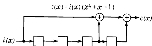
Рис. 6.13. Несистематический кодер для (15, 11)-кода Хэмминга.
