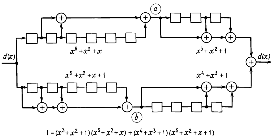
Рис. 12.11. Подробная схема регистра сдвига.
