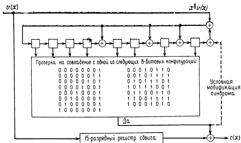
Рис. 6.22. Декодер Меггитта для (15, 7)-кода БЧХ.
