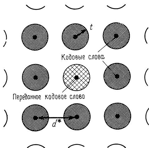
Рис. 14.2. Области декодирования.
