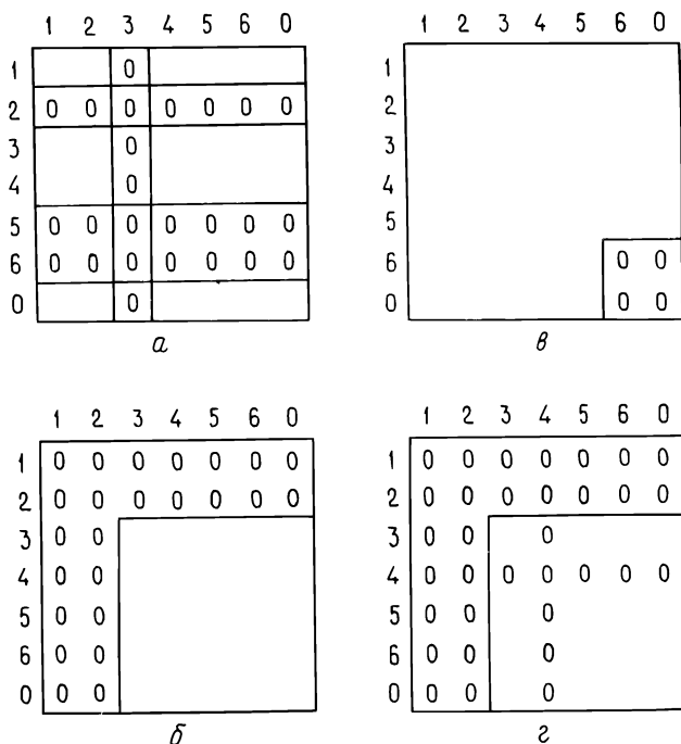
Рис. 10.4. Спектры некоторых кодов над GF(8) . a — произведение циклических кодов; б — произведение кодов Риды—Соломона; в — дуальный код-произведение; г — произведение (7, 4)-кодов БЧХ.
