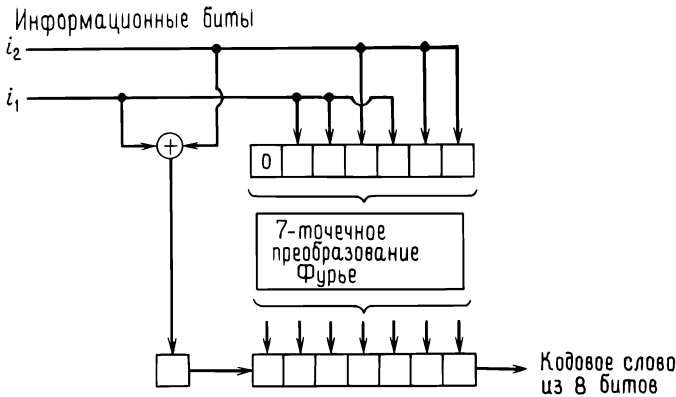
Рис. 8.12. Кодер для (8, 2, 5) -кода Гоппы.
