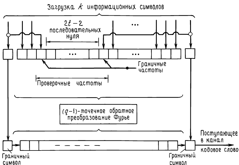
Рис. 8.6. Кодер для расширенного кода Рида—Соломона в частотной области.
