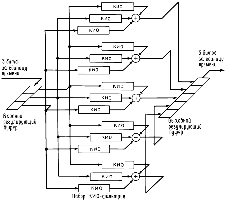
Рис. 12.8. Сверточный кодер ( n_0 = 5 , k_0 = 3 ).
