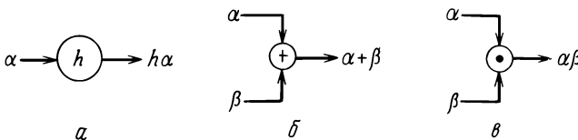
Рис. 6.2. Элементы устройств. a — умножитель на скаляр; б — сумматор, в — умножитель.
