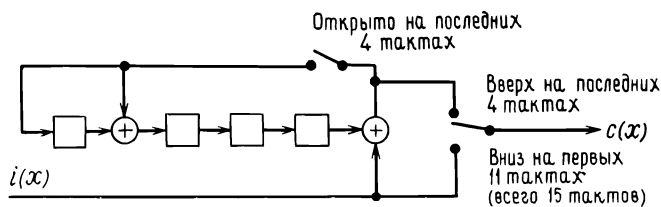
Рис. 6.16. Другой систематический кодер для (15, 11)-кода Хэмминга.
