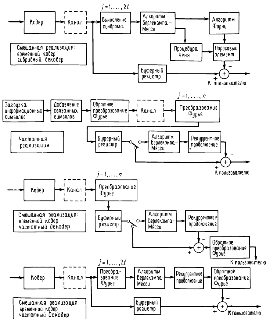
Рис. 9.2. Некоторые схемы кодера/декодера для кодов БЧХ.
