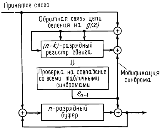
Рис. 6.20. Другой декодер Меггитта.
