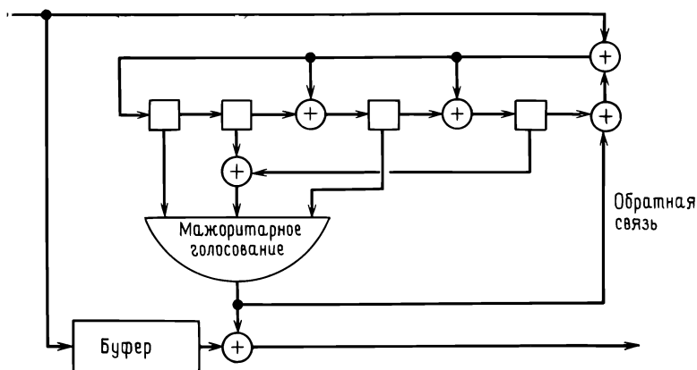
Рис. 13.2. Декодер Меггитта для симплексного (7, 3)-кода.
