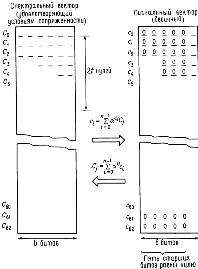
Рис. 8.3. Кодирование кодом БЧХ с помощью преобразования Фурье.
