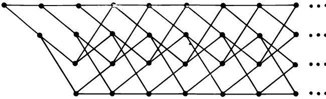
Рис. 12.4. Решетка сверточного кода
