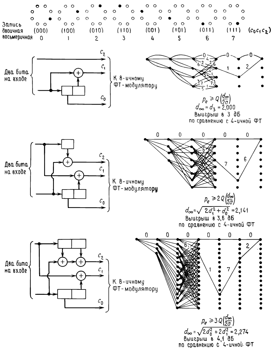
Рис. 15.8. Некоторые коды для восьмеричного канала с ФТ-модуляцией.
