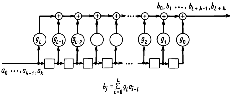
Рис. 6.9. Регистр сдвига без обратной связи.
