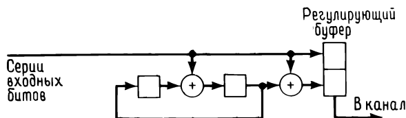
Рис. 12.10. Систематический кодер с обратной связью для сверточного (6, 3)-кода.
