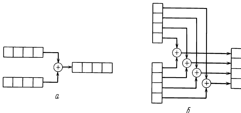
Рис. 6.4. Сложение двух элементов поля. a — последовательное исполнение; б — параллельное исполнение.
