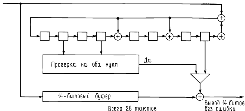
Рис. 6.29. Декодер с вылавливанием ошибок для кода-перемежения, исправляющего пакеты ошибок,
