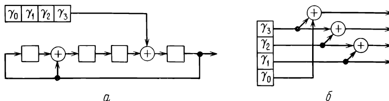
Рис. 6.5. Умножение на константу поля \beta = z^3 . a — последовательное исполнение; б — параллельное исполнение.
