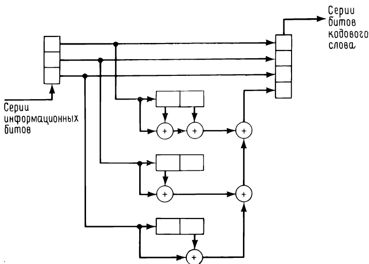
Рис. 12.12. Кодер для (12, 9) -кода Вайнера—Эша.
