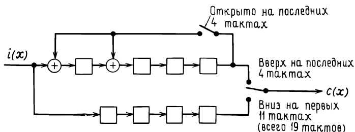
Рис. 6.15. Систематический кодер для (15, 11)-кода Хэмминга.
