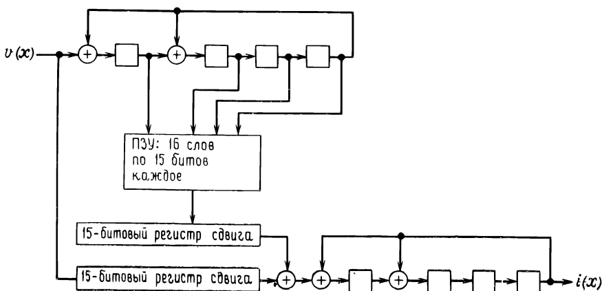
Рис. 6.17. Синдромный декодер для несистематического (15, 11)-кода Хэмминга.
