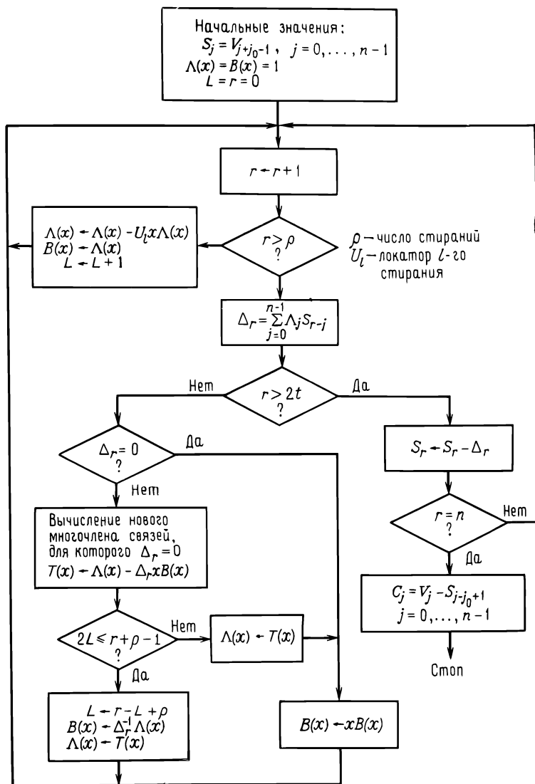
Рис. 9.4. Исправляющий ошибки и стирания декодер для кодов БЧХ.
