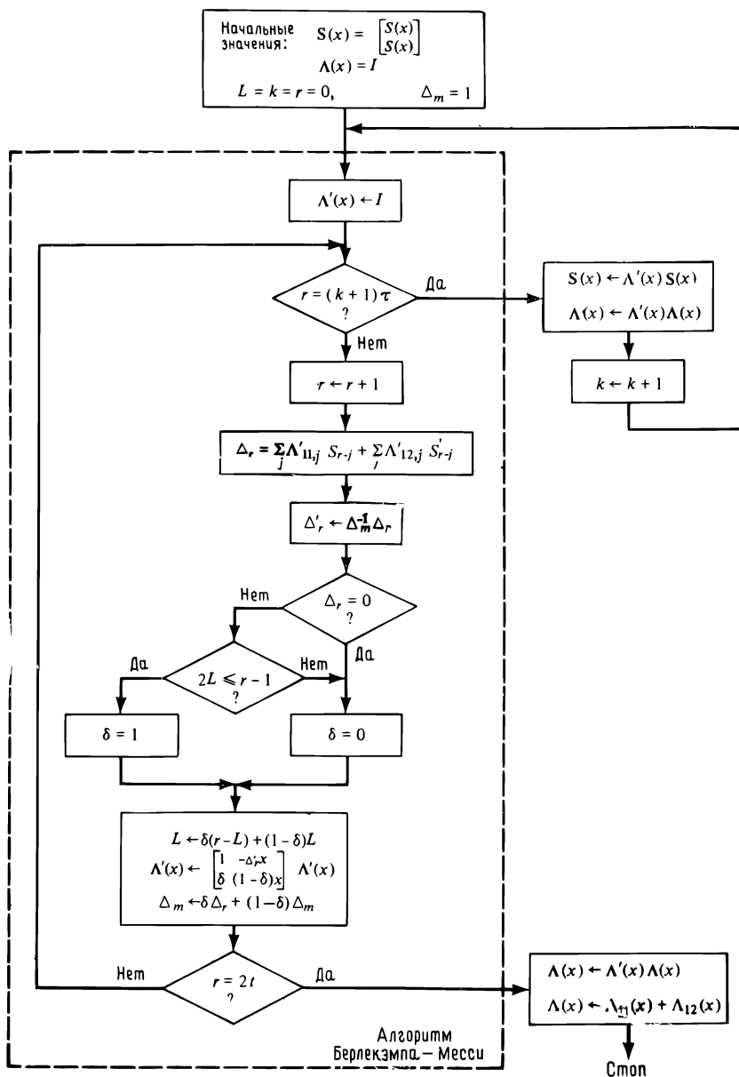
Рис. 11.7. Ускоренный алгоритм Берлекэмпа—Мессис.
