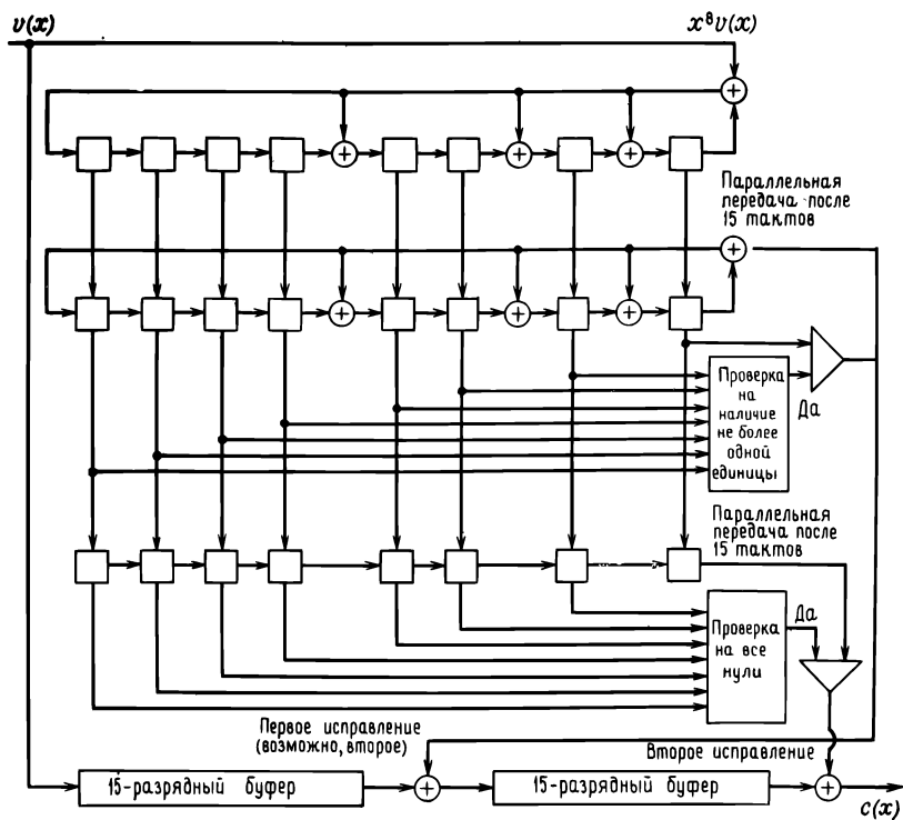
Рис. 6.25. Конвейерный вариант декодера с вылавливанием ошибок для (15, 7)-кода БЧХ.
