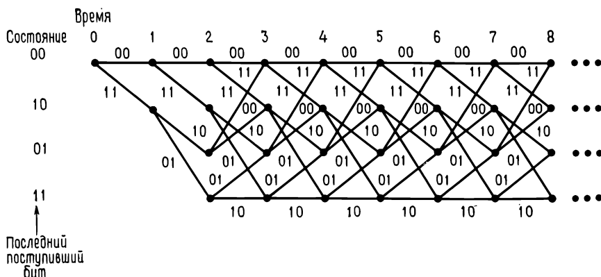
Рис. 14.4. Представление сверточного (6, 3)-кода с помощью решетки.
