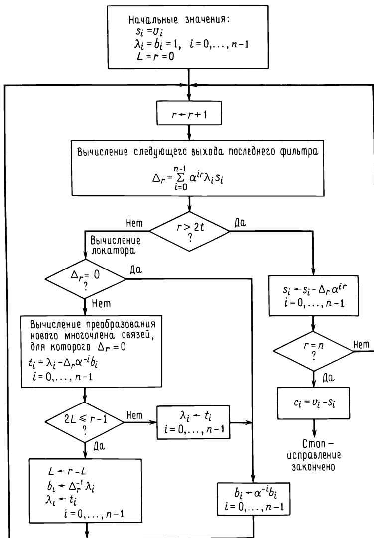
Рис. 9.7. Временной декодер.
