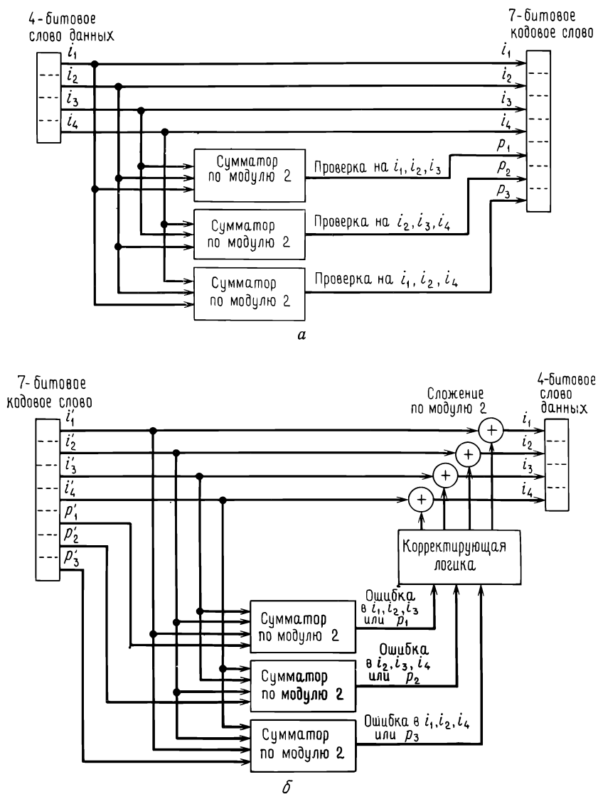
Рис. 1.4. Кодер/декодер для простого (7, 4)-кода Хэмминга. а — кодер; б — декодер.
