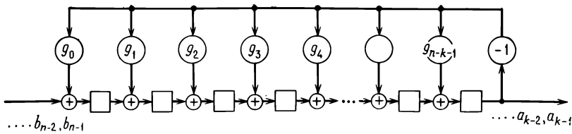
Рис. 6.11. Устройство деления на многочлен g(x) .
