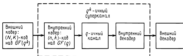
Рис. 7.9. Каскадное кодирование.
