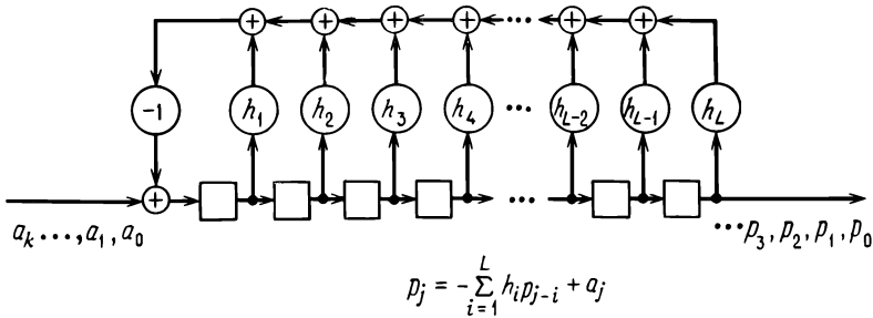
Рис. 6.8. Авторегрессионный фильтр.
