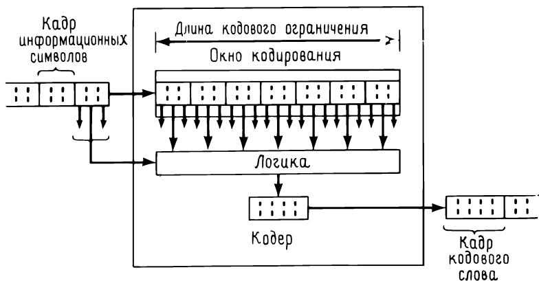
Рис. 12.1. Кодер в виде регистра сдвига,
