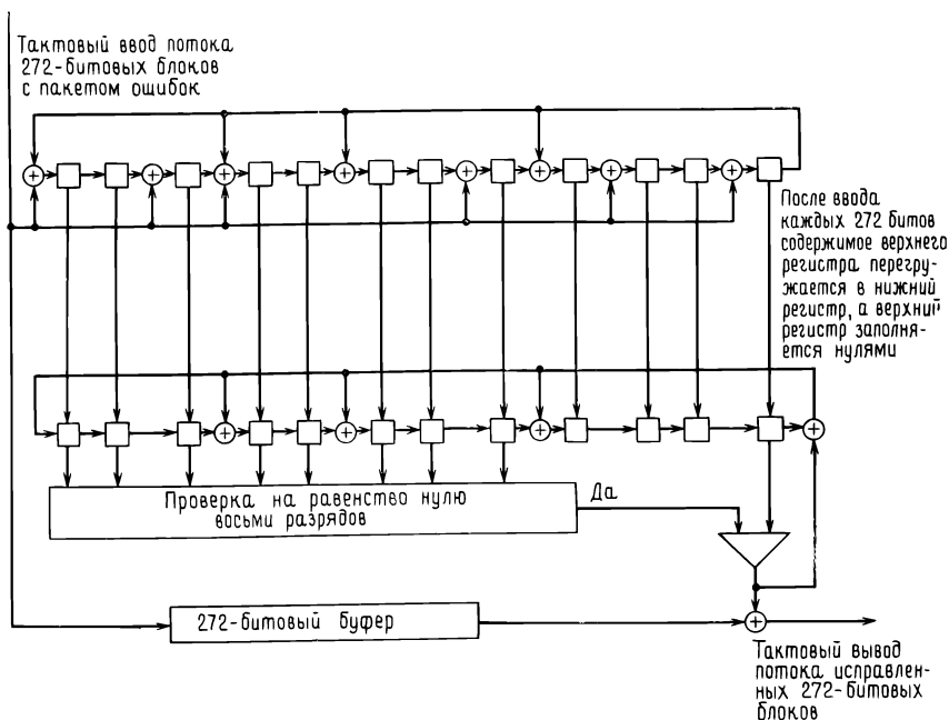
Рис. 6.30. Декодер с вылавливанием ошибок для (272, 260)-кода, исправляющего пакеты ошибок.
