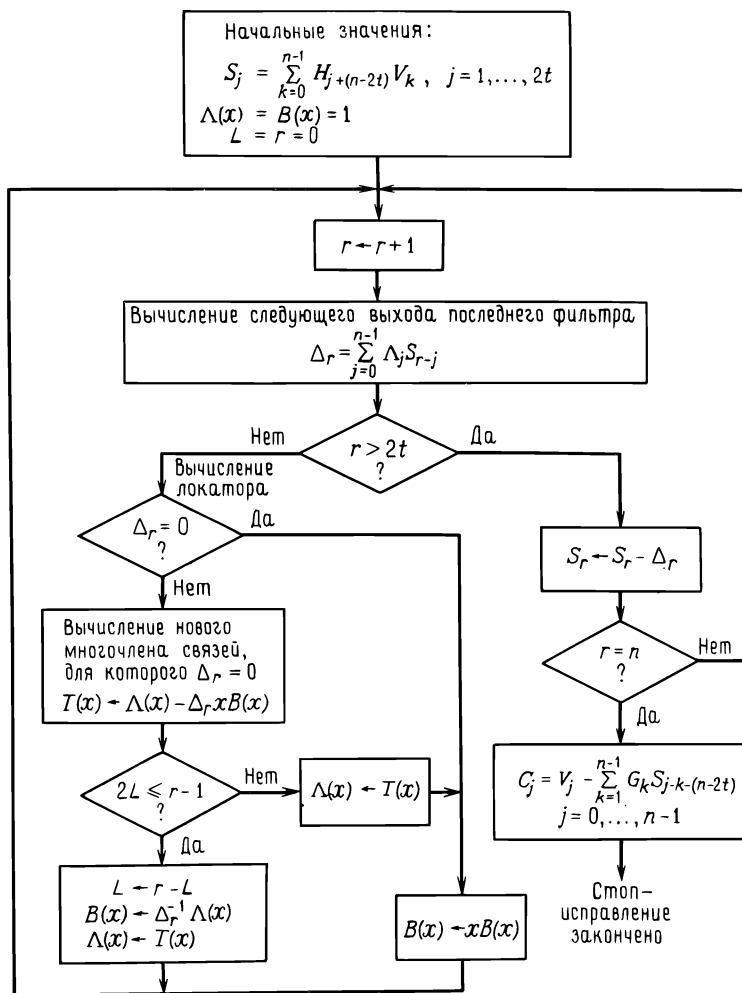
Рис. 9.8. Декодер для альтернантного кода.
