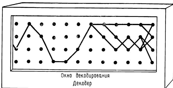
Рис. 12.24. Наглядное представление работы декодера Витерби.
