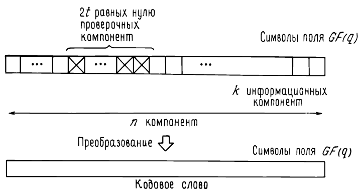
Рис. 8.2. Кодирование кодом Рида—Соломона с помощью преобразования Фурье.
