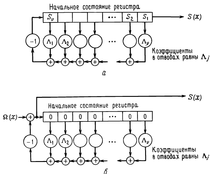
Рис. 7.4. Генерация спектра ошибок. a — вариант Мессси; b — вариант Берлекэмпа.
