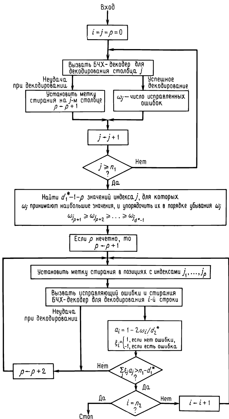
Рис. 10.2. Декодер для кода-произведения кодов БЧХ.
