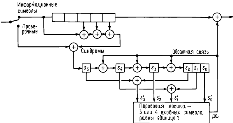
Рис. 13.4. Мажоритарный декодер для сверточного (12, 6)-кода.
