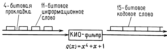
Рис. 6.14. Кодирование длинного потока битов.
