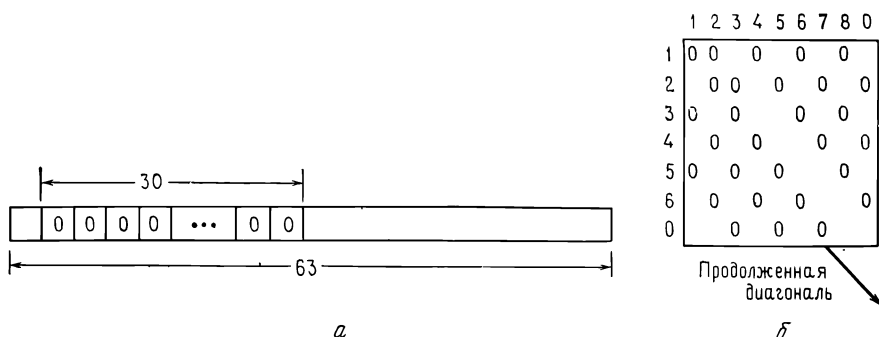
Рис. 10.6. Спектр быстрого кода БЧХ. a — спектр (63, 33, 31)-кода Риды—Соломона; б — двумерный спектр быстрого (63, 33, 31)-кода Риды—Соломона,
