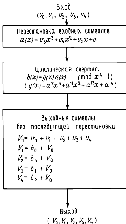
Рис. 9.10. Вычисление пятиточечного преобразования Фурье с помощью алгоритма Рейдера.
