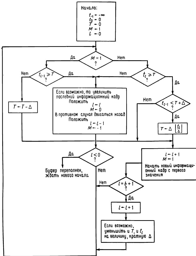
Рис. 12.28. Алгоритм Фано.
