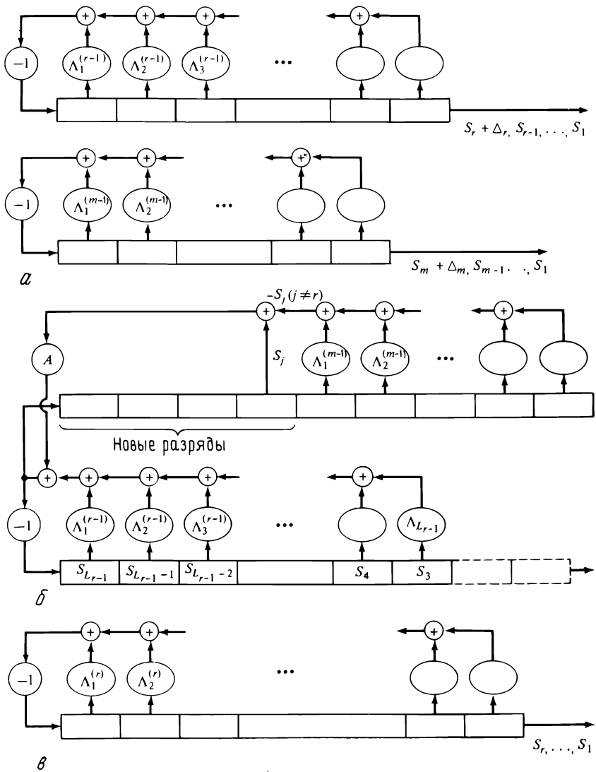
Рис. 7.3. Конструкция Берлекэмпа—Мессе.
