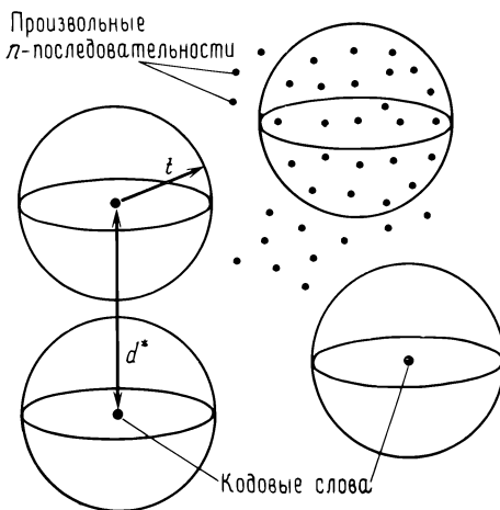
Рис. 1.3. Сферы декодирования.
