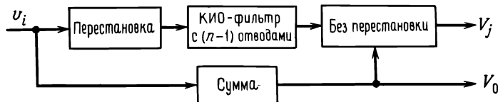
Рис. 9.9. Переход от преобразования Фурье к свертке.
