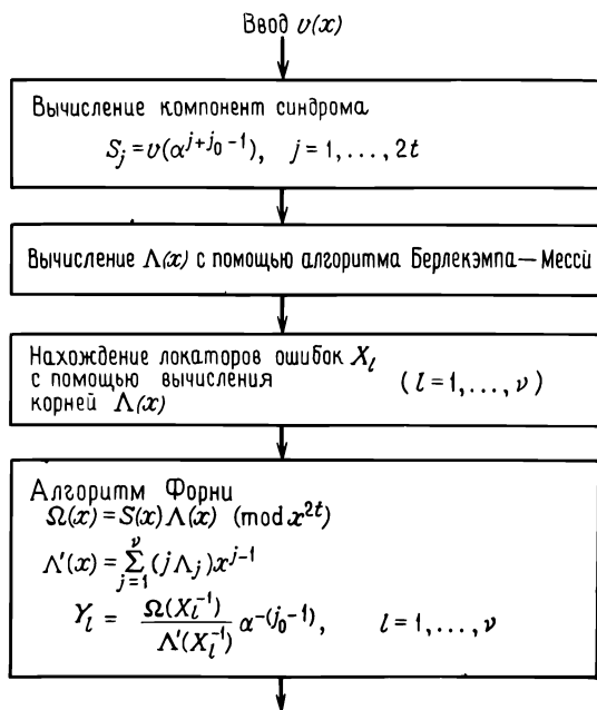
Рис. 7.7. Быстрое декодирование кодов БЧХ.
